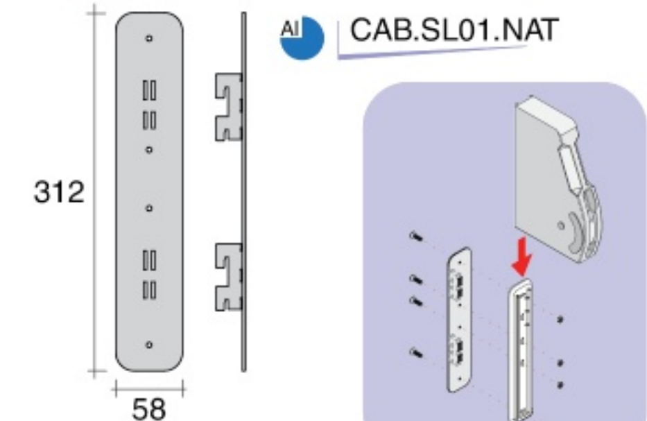
Einzelnes Wandelement LIFT für doppelte Schlitzschiene
