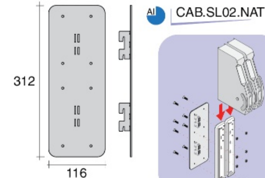
Doppeltes Wandelement LIFT für doppelte Schlitzschiene
