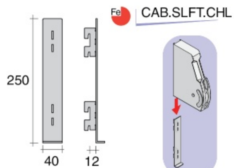
Einzelnes Wandelement LIFT für Schlitzschiene
