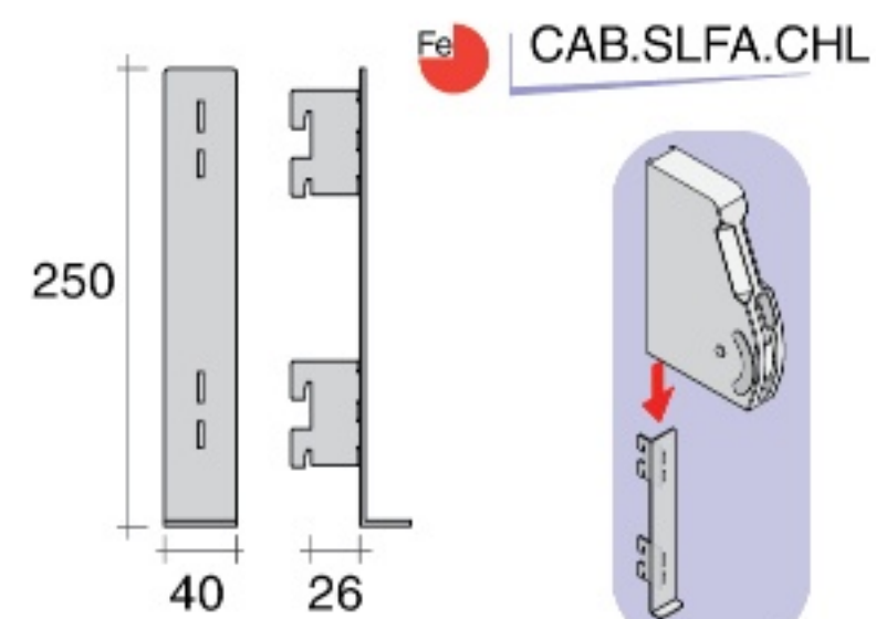
Einzelnes Wandelement LIFT für Schlitzschiene mit Distanzstück kombinierbar mit CAB.SL02.NAT
